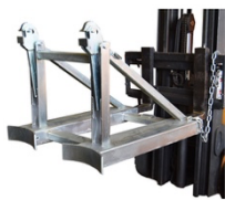
Pince à fûts galvanisée 720 kg
