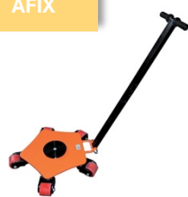
Rouleur pivotant 2 à 4 t
